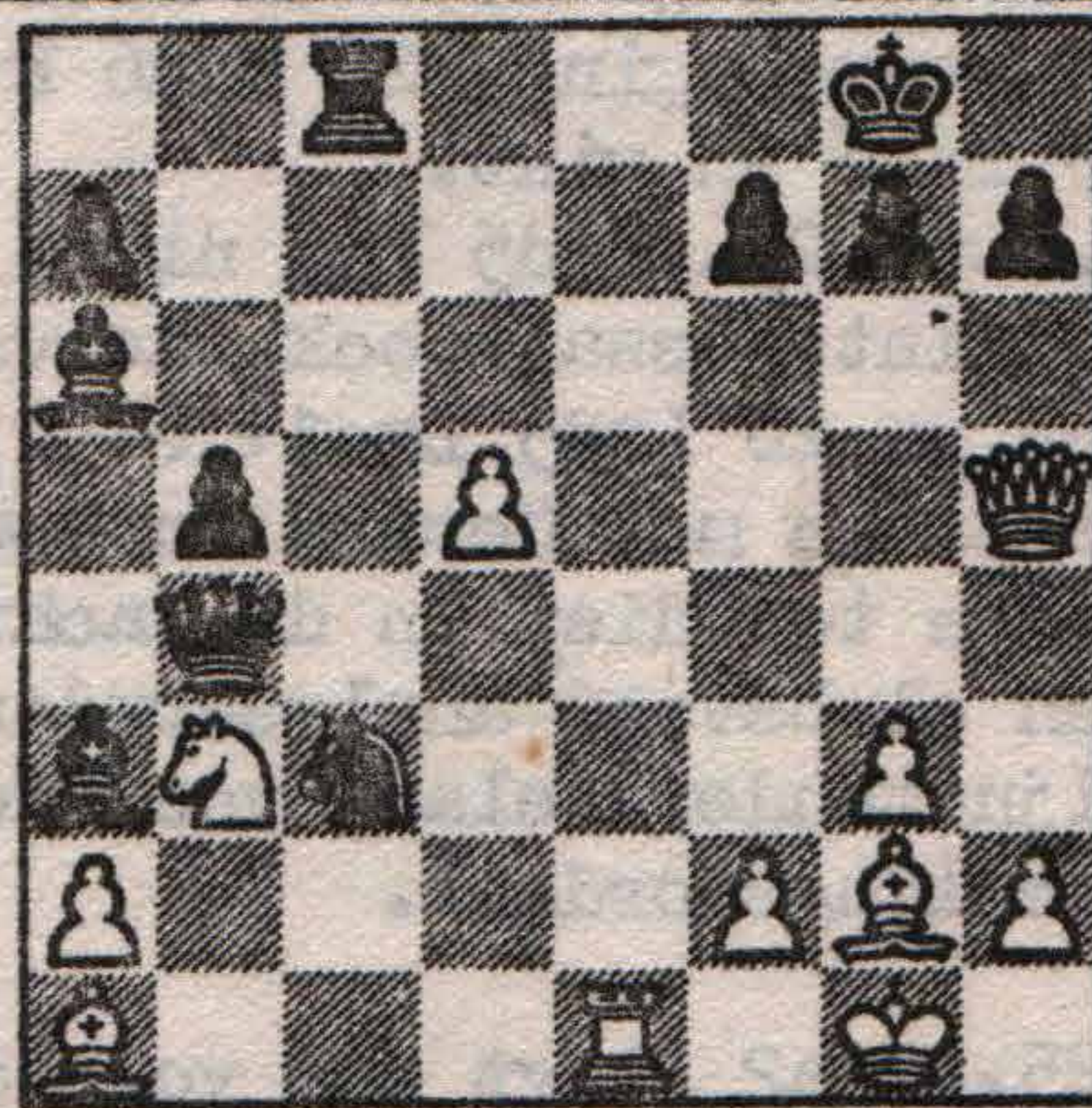
Diagram na 25 Dh5 !
