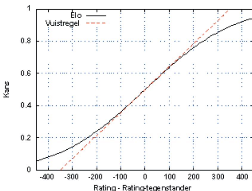
Figuur 3: Verwachte score volgens Elo en de benadering van deze kromme met een rechte lijn
