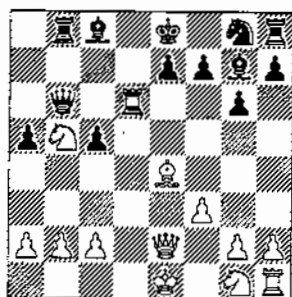
Krassilnikov-Beckmann
